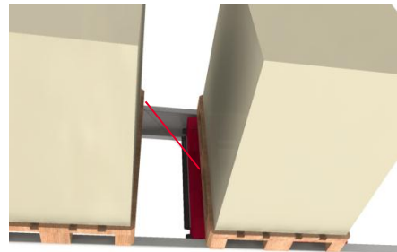
Sensores de acercamiento a palés para su correcto posicionamiento
